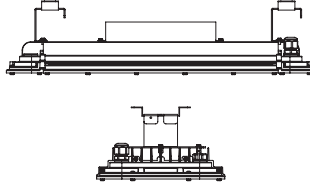
Kablo Tavası ve Tavan Bağlantı Aparatı
